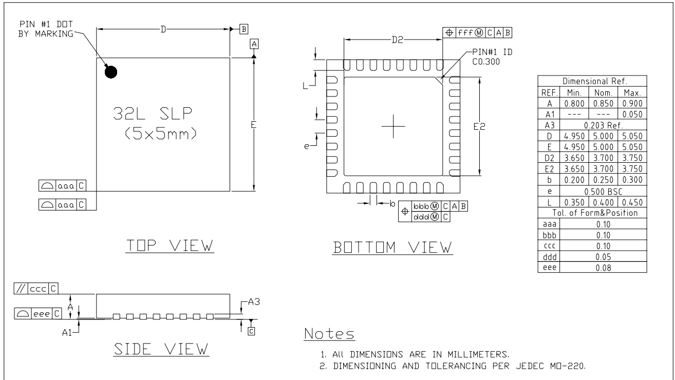
图 5-1. QFN32 (5x5 mm) 封装
