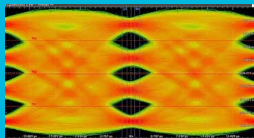
在带有 TSO8C18 光模块的泰克 TSO820 采样示波器上采集的 53Gb/s PRBS15Q 信号的示例，由 TCR801 光学时钟恢复触发
