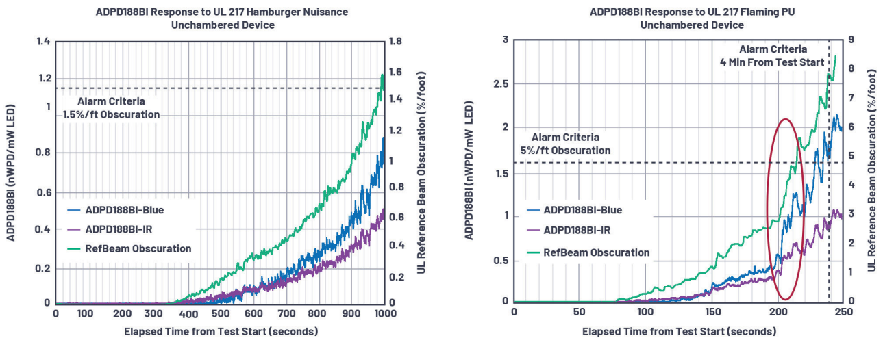
图3. ADPD188BI UL测试结果：在无烟室中进行汉堡烟雾和易燃聚氨酯烟雾检测。
