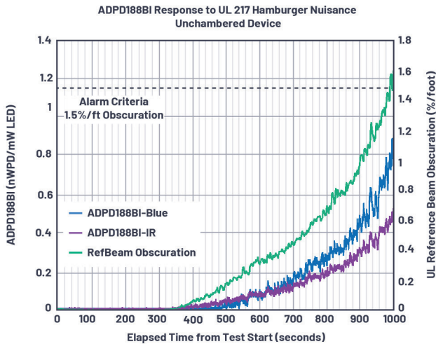
图3. APDPD188BI UI测试结果：在无烟室中进行汉堡烟雾和易燃聚氨酯烟雾检测。
