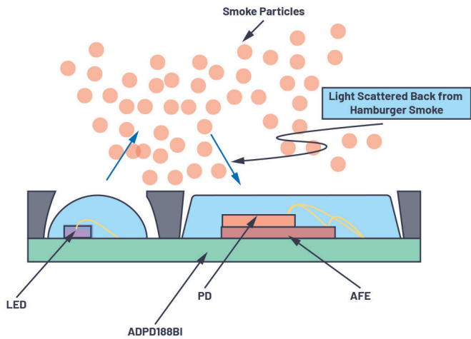
图2. ADPD188BI的工作原理。
